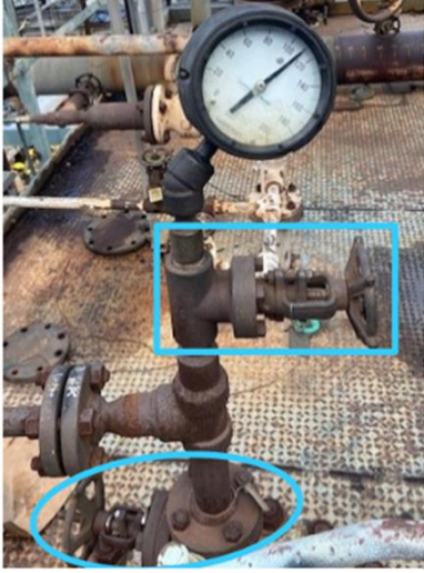
شکل 1۔ والوز ء الگ کنگ ء انت پریشر گنج
